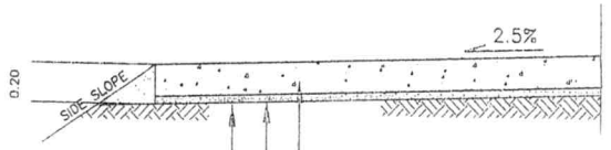
รูปตัดแฉัดโครงสร้างถนนคอนกรีตเสริมเหล็กและคูมลิมป์ตีวัลดู มาตรฐาน
