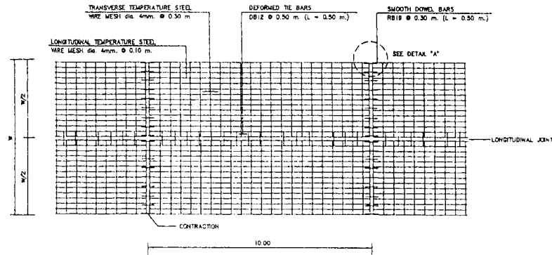
แบบแสดงการเสริมเหล็ก ถนน ค.ล.ล
