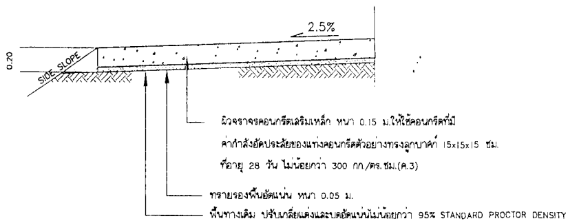
รูปตัดขยายขึ้นโครงสร้างทาง มาตรฐาน
